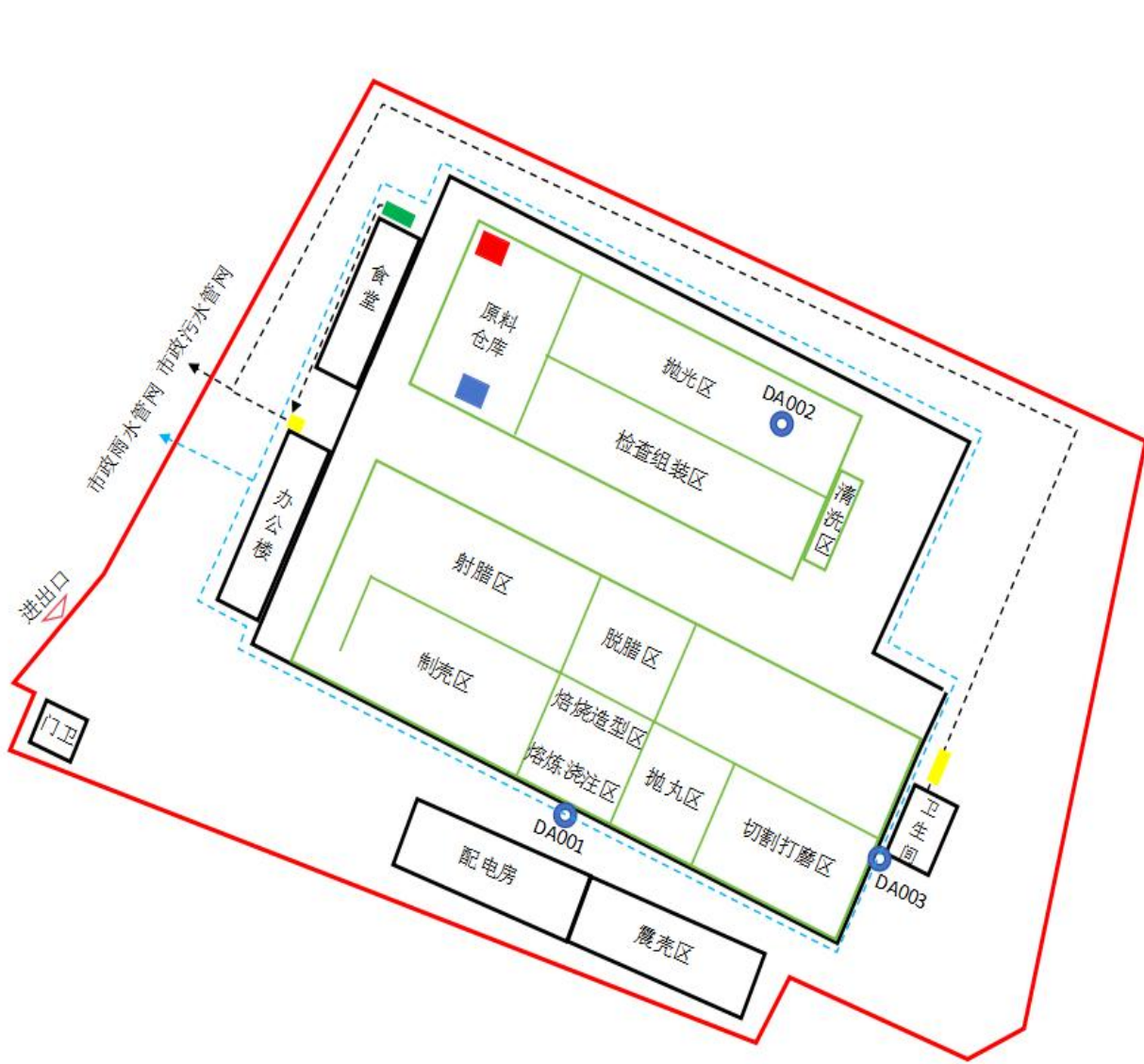
附图3 项目总平面布置图及雨污管网图
